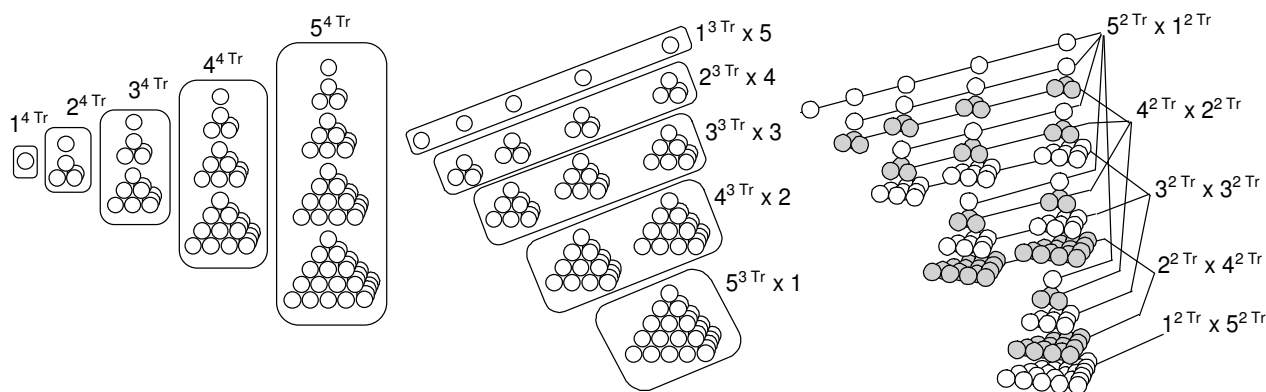
Рисунок 3-14. Множественность группировок одних и тех же элементов для 5^5\text{Tr} = 126 .
