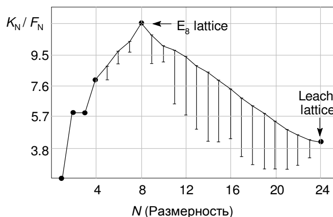
Рисунок 3-5. Зависимость верхних пределов K_N / F_N от N .
