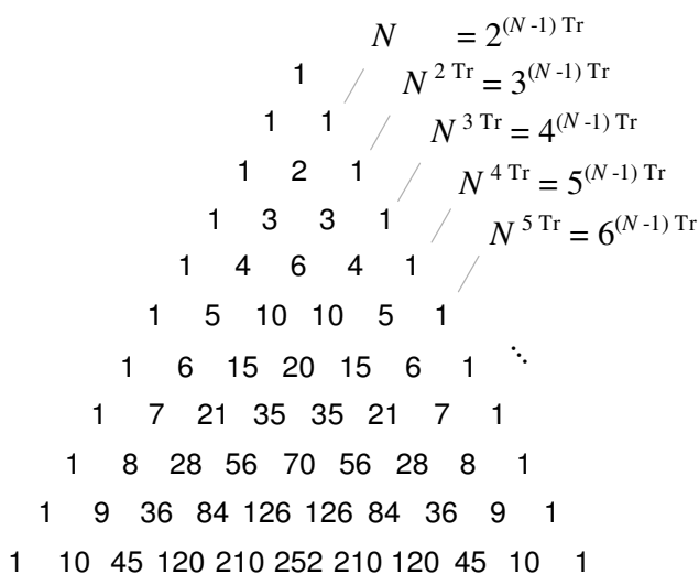
Рисунок 3-20. Треугольник Паскаля до десятой строчки
