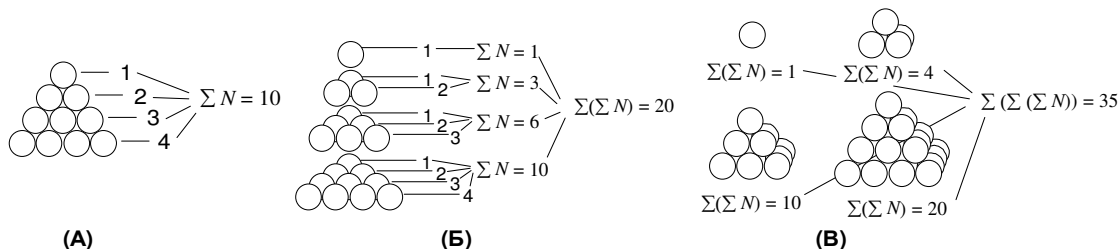
Рисунок 3-19. Образование треугольных чисел N^2 \text{Tr} (А), тетраэдрических чисел N^3 \text{Tr} (Б), и пентатопных чисел N^4 \text{Tr} (В).
