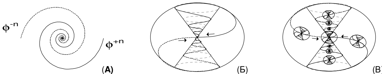
Рисунок 4-5. Двойная логарифмическая спираль (А) порождает логарифмический вихрь (Б), который есть часть более сложной системы (В)
