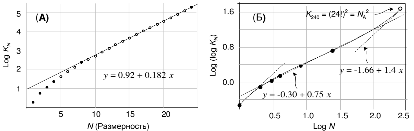
Рисунок 3-4. Зависимость верхних пределов K_N от N .
