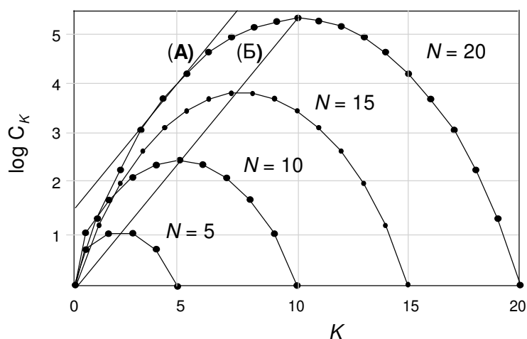
Рисунок 3-21. Зависимость чисел в Треугольнике Паскаля ( C_K ) от их позиции в строке ( K ).
