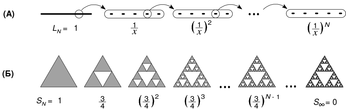
Рисунок 2-2. Примеры фрактальности.
