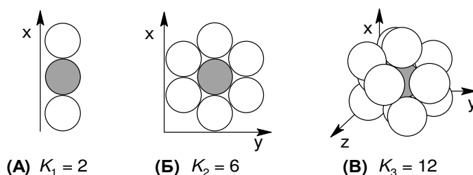
Рисунок 3-1. Иллюстрация понятия K_N для N = 1, 2, \text{ и } 3
