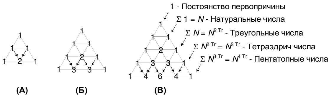
Рисунок 3-18. Образование Треугольника Паскаля
